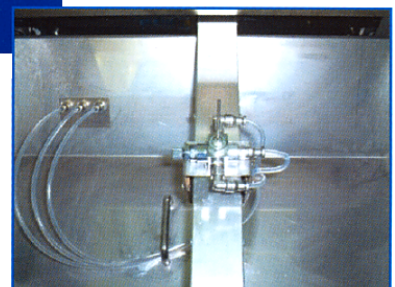
低圧ニードル式噴霧ノズル
